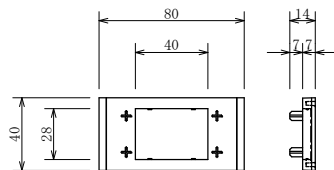
反射板取付プレート詳細図
