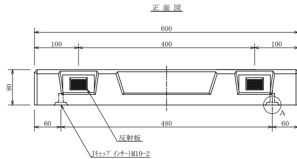
反射板取付プレート詳細図
