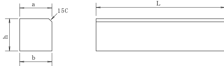
地先境界ブロック
