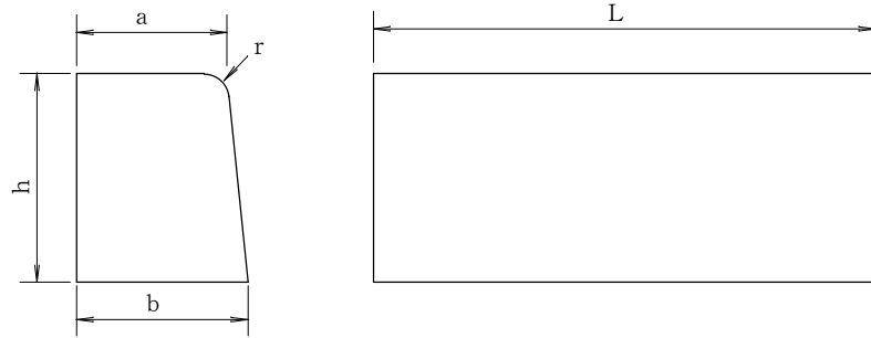
片面歩車道境界ブロック
