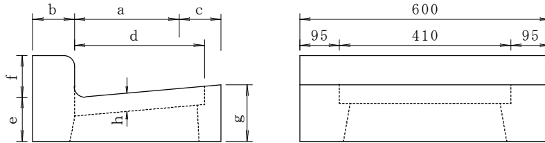
寸法表
