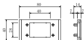
反射板取付プレート詳細図
