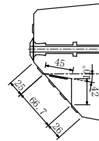
A-A 矢視詳細図
