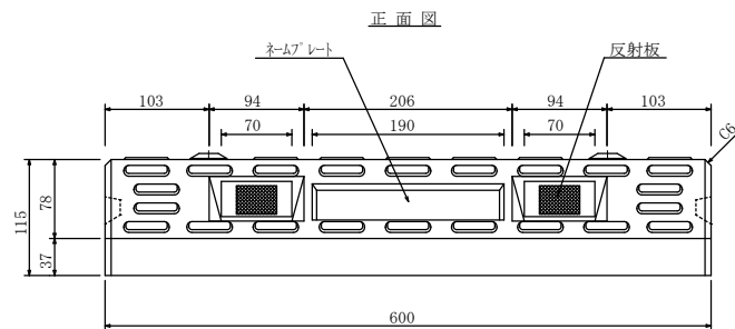
反射板取付プレート詳細図
