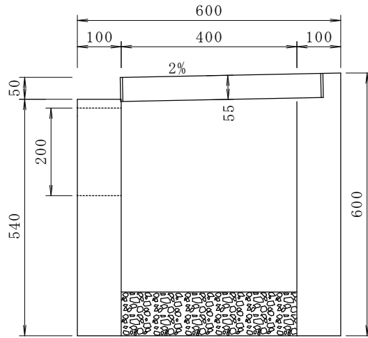
側面図
