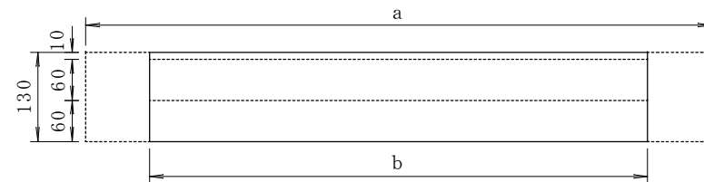
正面図
