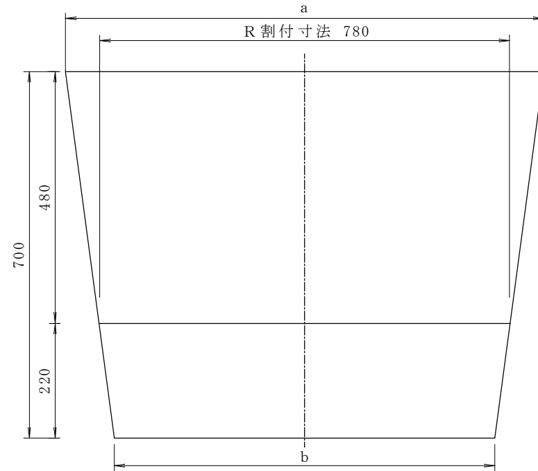
平面図
