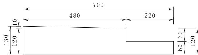
側面図
