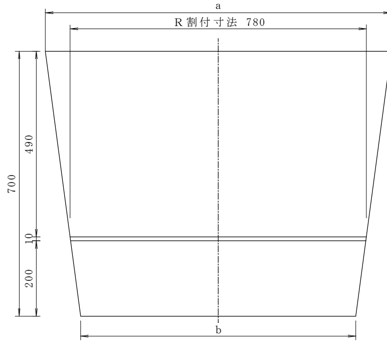
正面図
