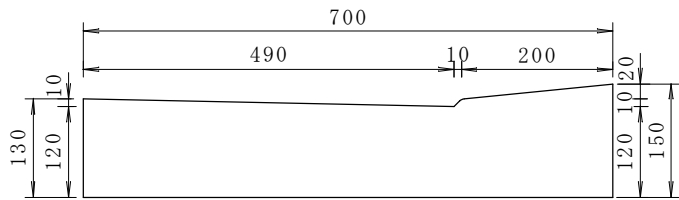
側面図
