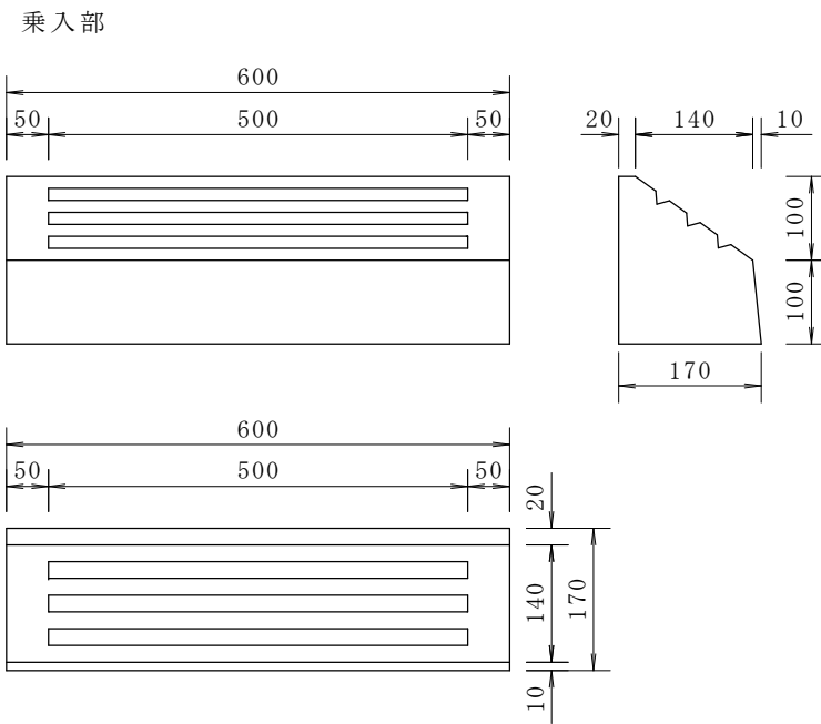
スリップ止め詳細
