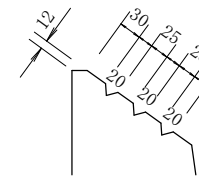
スリップ止め詳細
